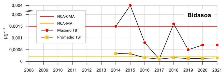
Figure 38 : Evolution des teneurs en TBT dans l'eau et comparaison avec les seuils dans l'eau (NCA-CMA : concentration maximale admissible et NCA-MA : concentration moyenne admissible) (Larreta et al. , 2022)
